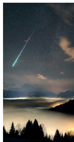
Geminiden 2023, Sternschnuppen und Feuerkugeln, Hermann Koberger, AAS
