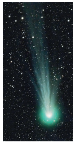
Komet Pons-Brooks war im April über Österreich zu sehen. Josef Hager, AAS
